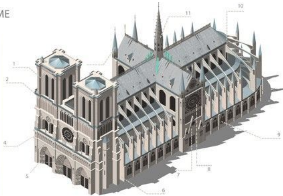
1. Torre; 2. Galería de las Quimeras; 3. Pináculo; 4. Galería de los reyes; 5. Pórtico central; 6. Contrafuerte; 7. Gablete; 8. Rosetón; 9. Vitrales; 10. Arbotante; 11. Aguja o flecha
